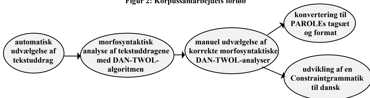
Figur 2: Korpussamarbejdets forløb
